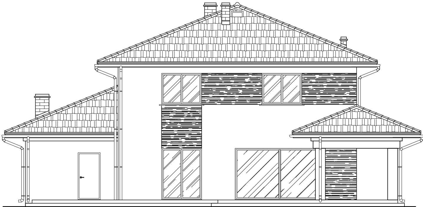
Elewacja tylna
